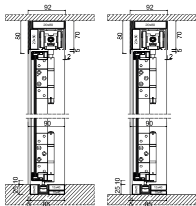
vertikaler Querschnitt (untere Schiene im Boden eingelassen)
