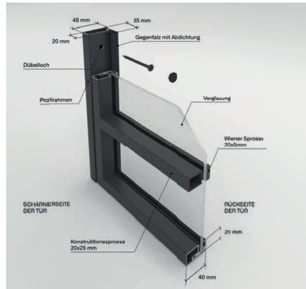
Rahmen- und Flügelquerschnitt mit Konstruktionssprosse
