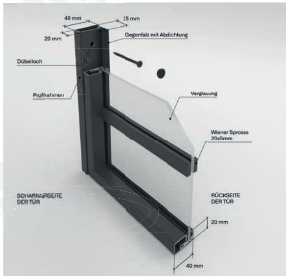
Rahmen- und Flügelquerschnitt mit Wiener Sprosse
