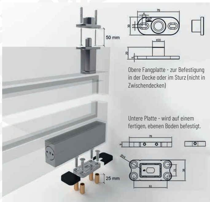
Montage des Argenta Pivotscharniers
